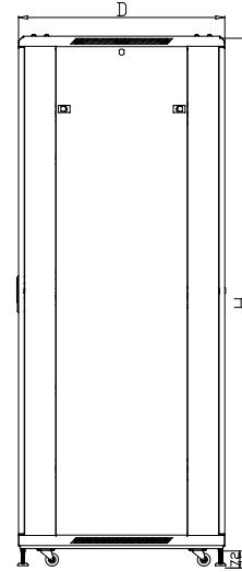
вид сбоку
